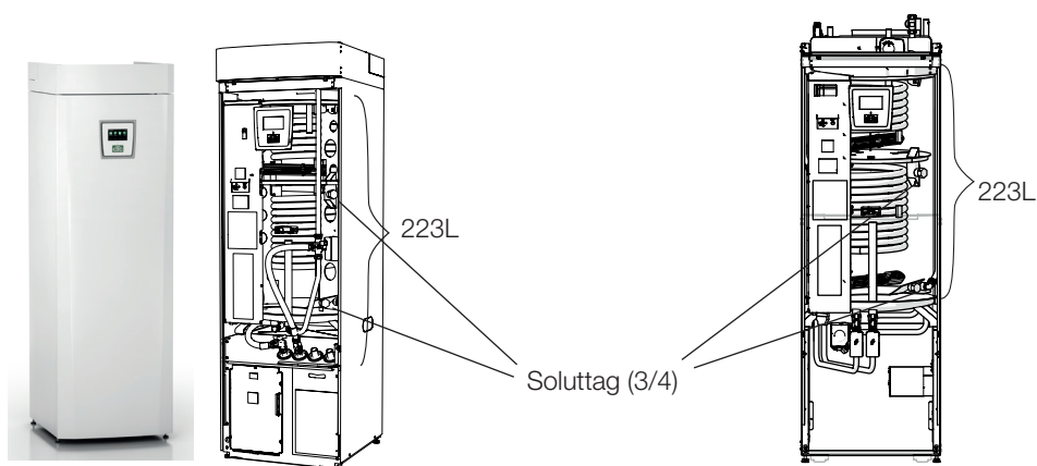
CTC Ecoheat 400 (223L med skiktskiva och soluttag).
