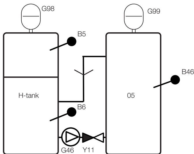
Principschema för difftermostatfunktion
